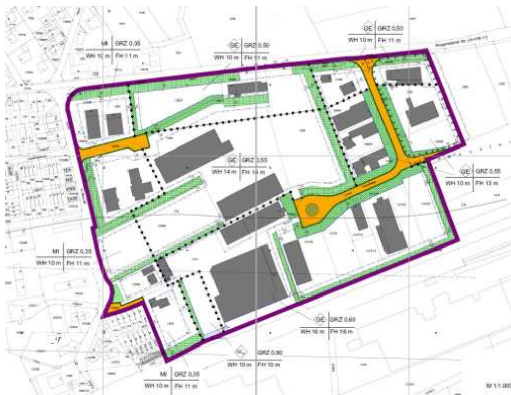
Abb.: Bebauungsplan Nr. 550 „Gewerbegebiet südlich der Roggensteiner Straße“, 4. Änderung, ohne Maßstab
